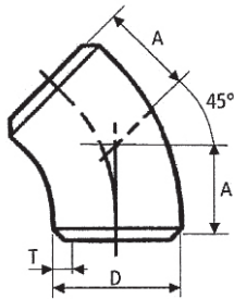
CURVE A SALDARE RICAVATA DA TUBO SALDATO DIMA 3 D - 45°
