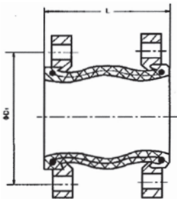
GIUNTO ANTIVIBRANTE CON FLANGE IN ACCIAIO ZINCATO 6002
