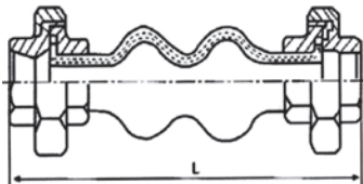
GIUNTO ANTIVIBRANTE FILETTATO 6001
